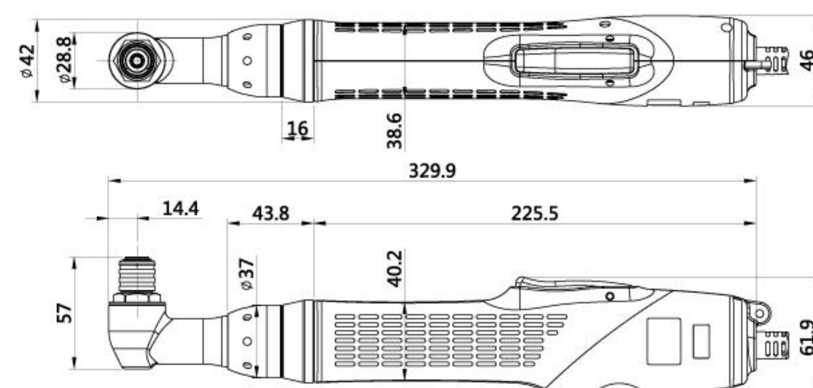
MY-SAVER 3 / 5 / 7 RA
