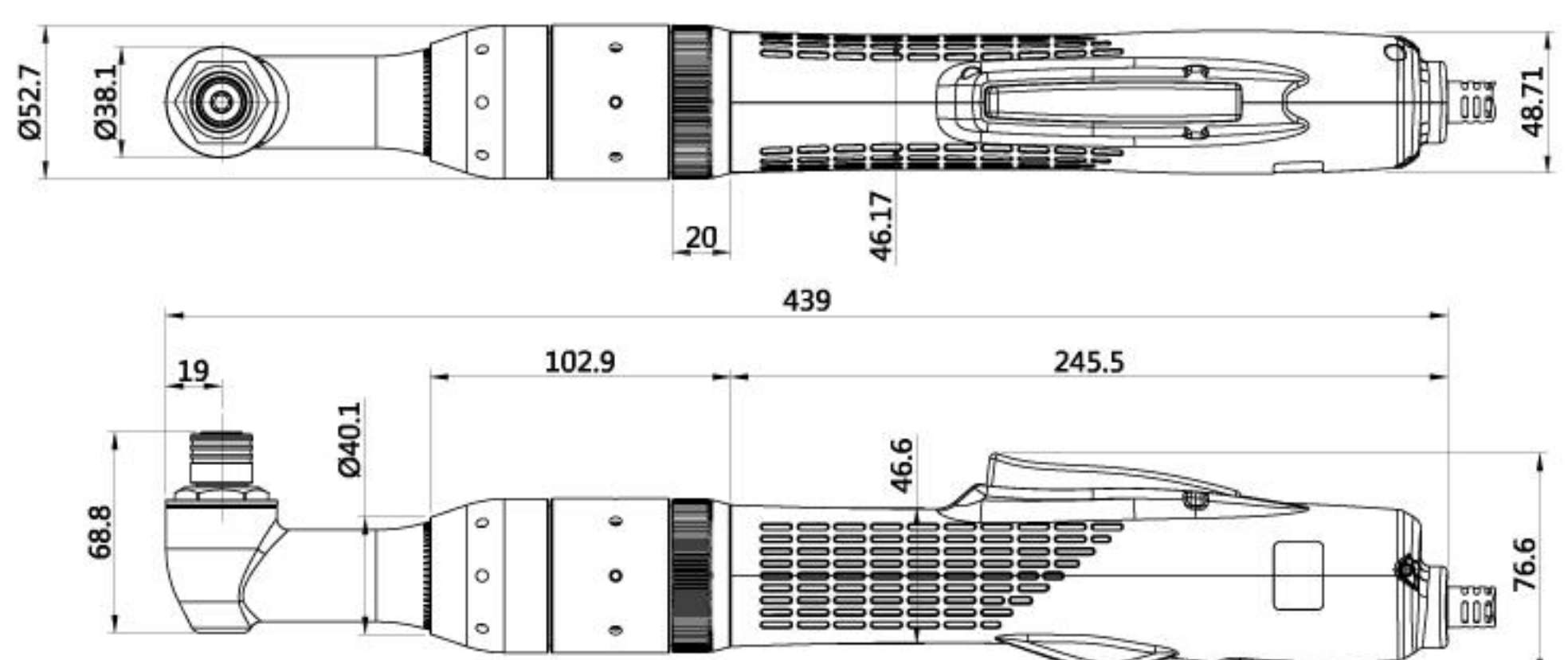
MY-SAVER 25 RA
