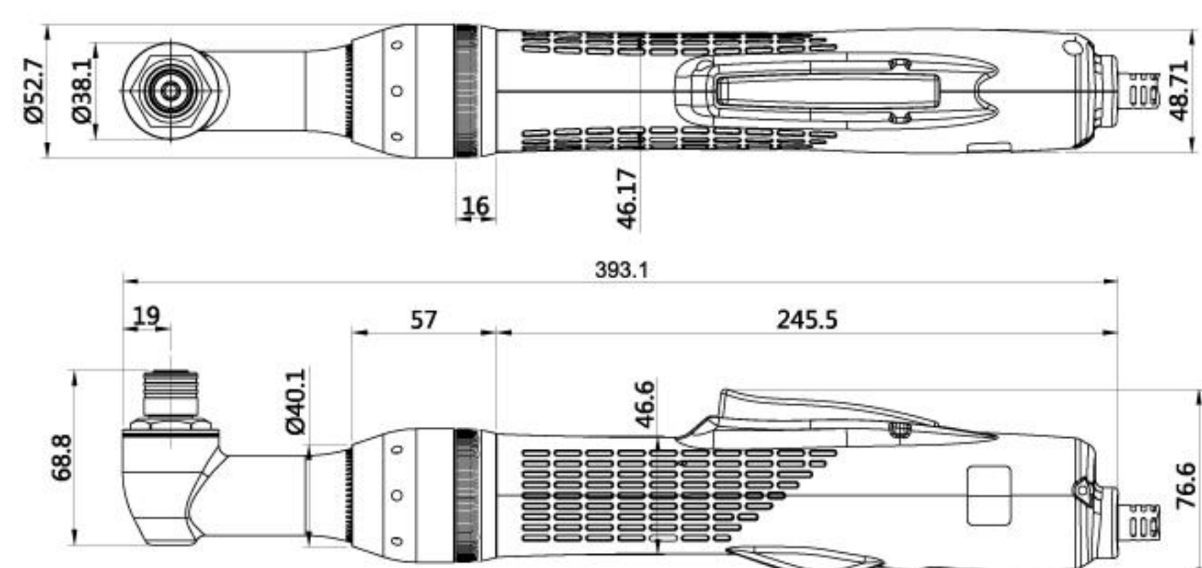
MY-SAVER 12 / 18 RA
